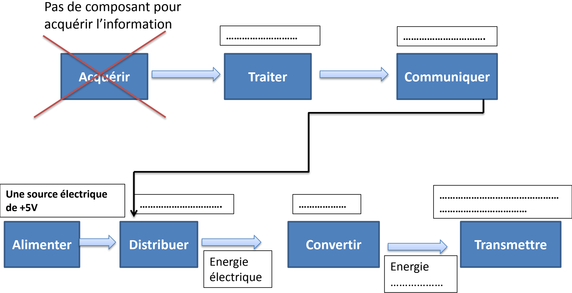
Chaîne fonctionnelle du signal S.O.S lumineux
