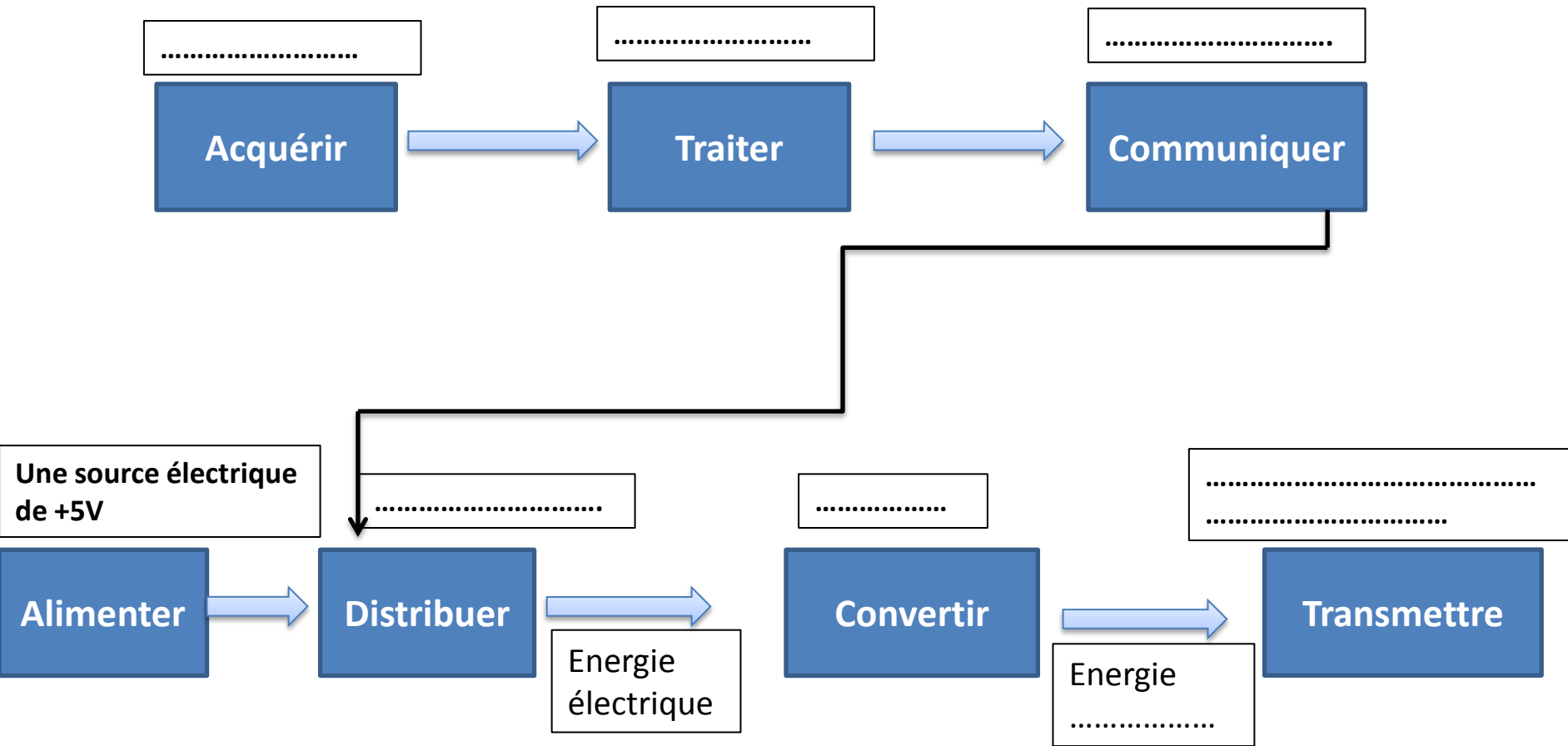
Chaîne fonctionnelle du système de détection
